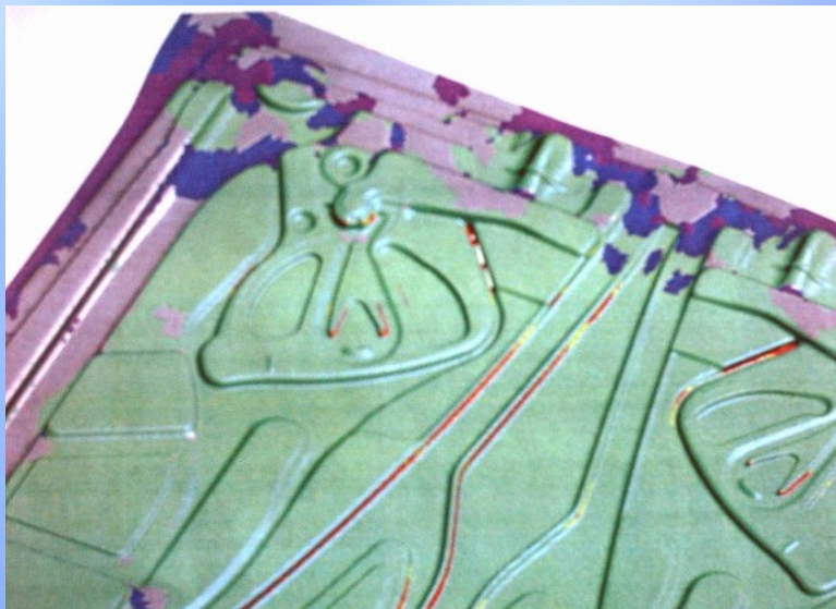
Material Aufbaurichtung des Bleches der RBT
